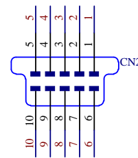
USB Mini Type B Male 10pin
