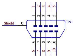
USB Mini Type B Female 10pin
